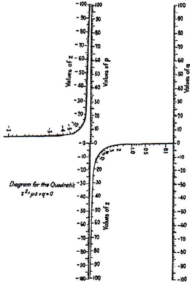
Figura 2. Solución de la ecuación cuadrática general [3].
