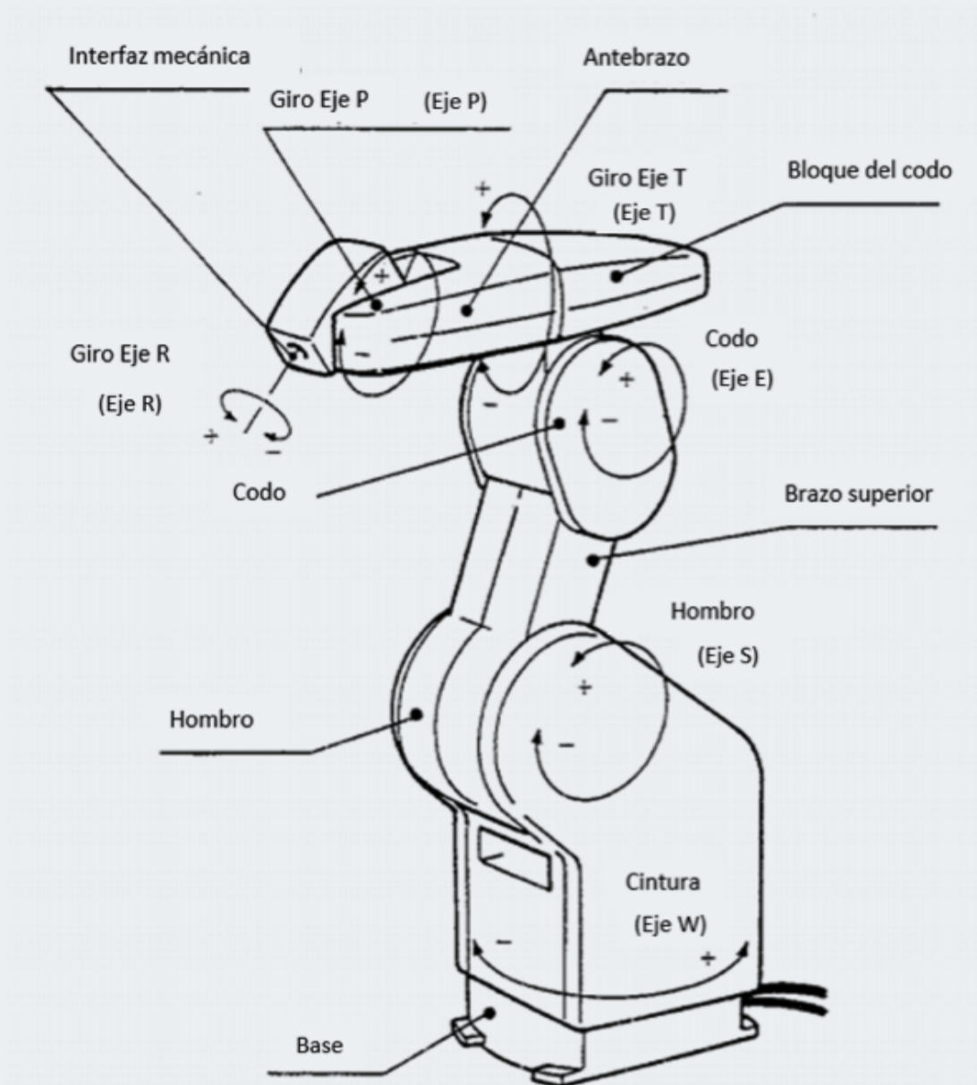
Figura 2. Partes y articulaciones del Robot Mitsubishi RV-E2
