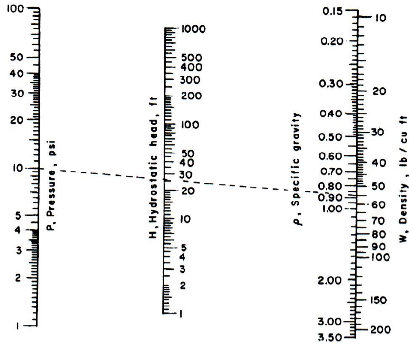
Figura 3. Cálculo de la cabeza hidrostática por la presión estática en un líquido [2].
