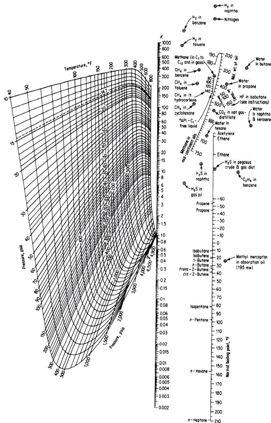
Figura 4. Constantes de equilibrio líquido-vapor de hidrocarburos [4].
